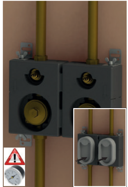
Montageschritt 3
