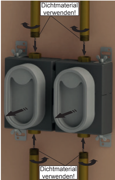
Montageschritt 4
